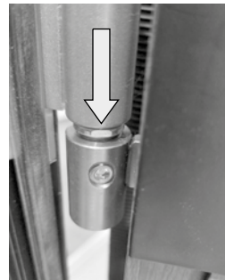
Fixierschraube lösen.
